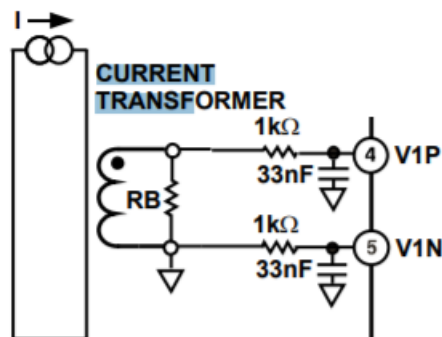
Figura 18 – Diagrama de utilização de transformadores de corrente. Fonte: Analog Devices (2010)
