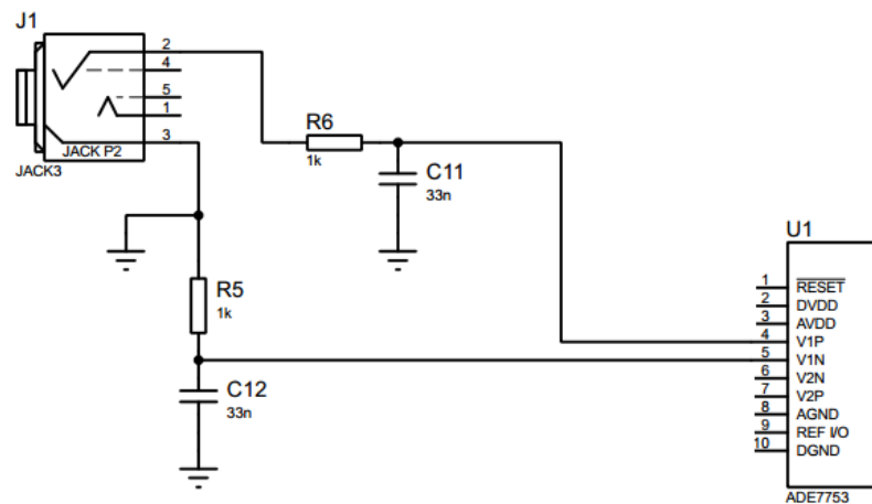
Figura 19 - Configuração de entrada do Canal 1 de Corrente
