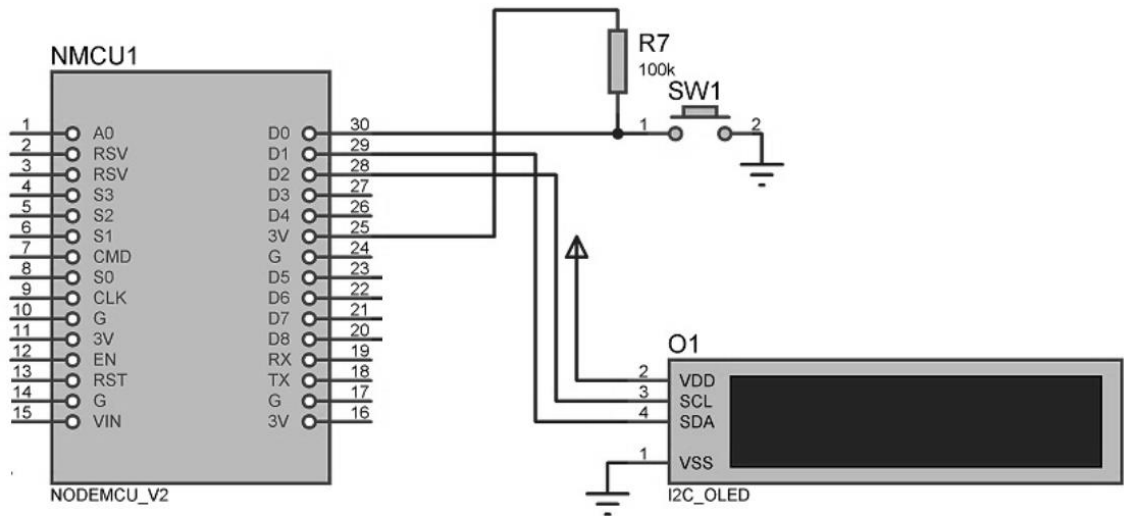
Figura 21 - Conexão do display OLED ao microcontrolador
