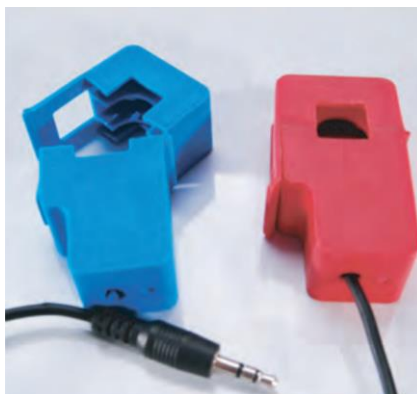
Figura 16 - Transformador de Corrente SCT-013-020. Fonte: Nice gear (2020)
