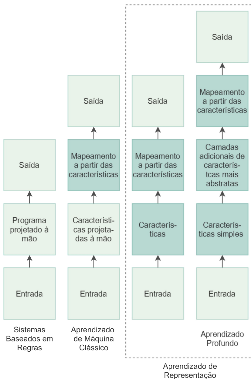
Figura 3 – Fluxograma que diferencia as áreas de estudo da Inteligência Artificial e suas etapas de processamento de dados.
