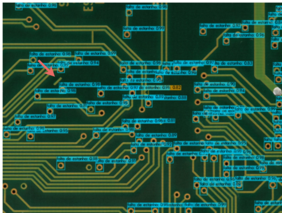
Figura 35 – Resultado de predição para imagem com defeito, teste 5.
