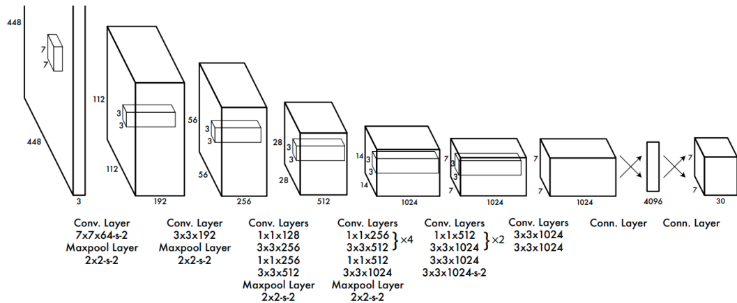
Figura 19 – Arquitetura da Rede Neural YOLO.
