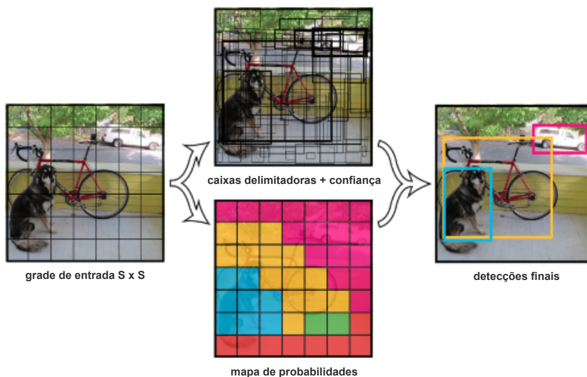
Figura 21 – Processo de detecção e classificação na rede neural YOLO.
