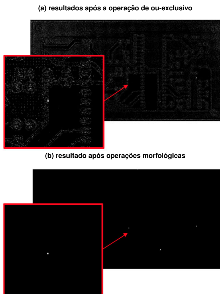
Figura 24 – Extração de defeitos em placas de circuito impresso utilizando métodos comparativos.
