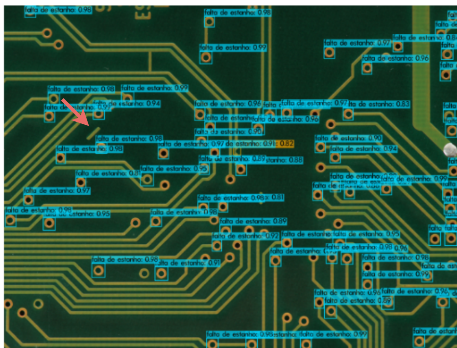
Figura 35 – Resultado de predição para imagem com defeito, teste 5.
