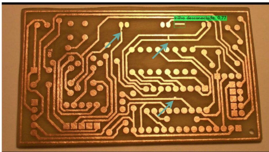
Figura 34 – Resultado de predição para imagem com defeito, teste 4.
