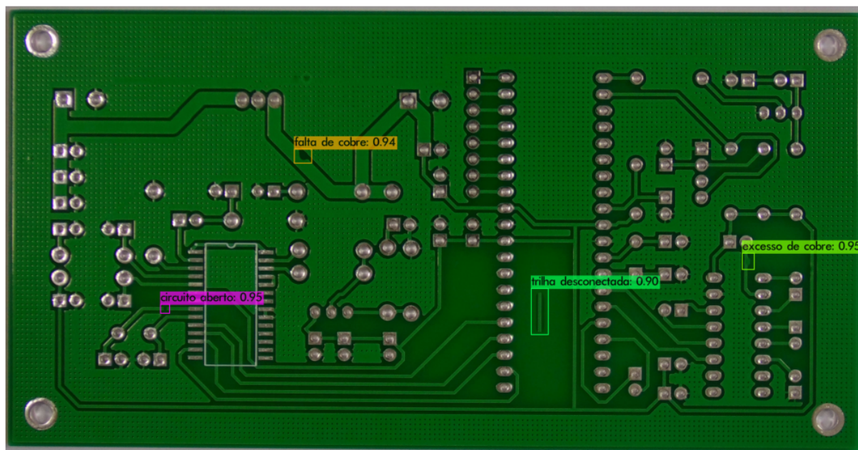
Figura 33 – Resultado de predição para imagem com defeito, teste 3.
