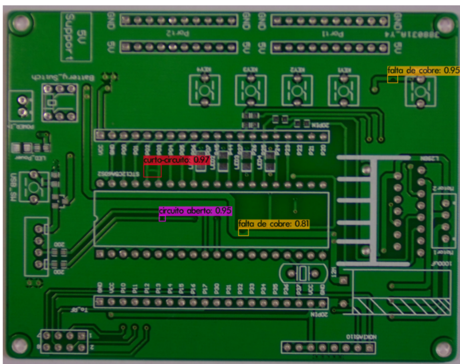
Figura 32 – Resultado de predição para imagem com defeito, teste 2.
