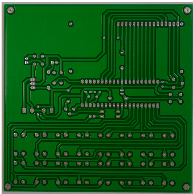
Figura 51 – PCI Número 12 do conjunto de dados HRIPCB.
