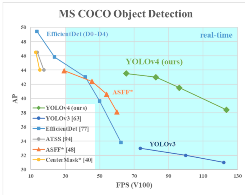
Figura 20 – Comparação da precisão média em função do processamento em frames por segundo para diferentes redes neurais utilizadas em detecção de objetos.
