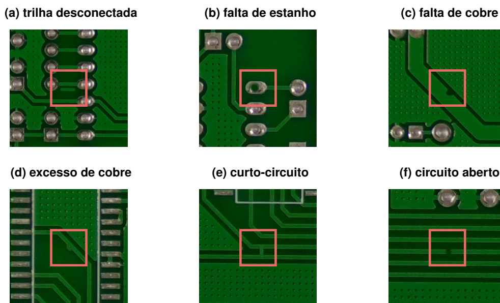
Figura 23 – Tipos de defeito de fabricação em placas de circuito impresso.
