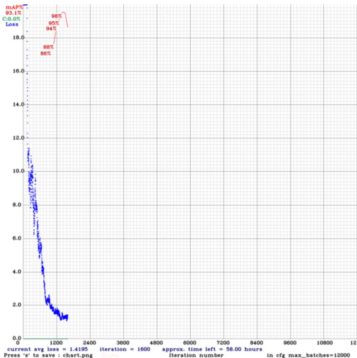
Figura 28 – Desempenho do início do treinamento da rede neural.
