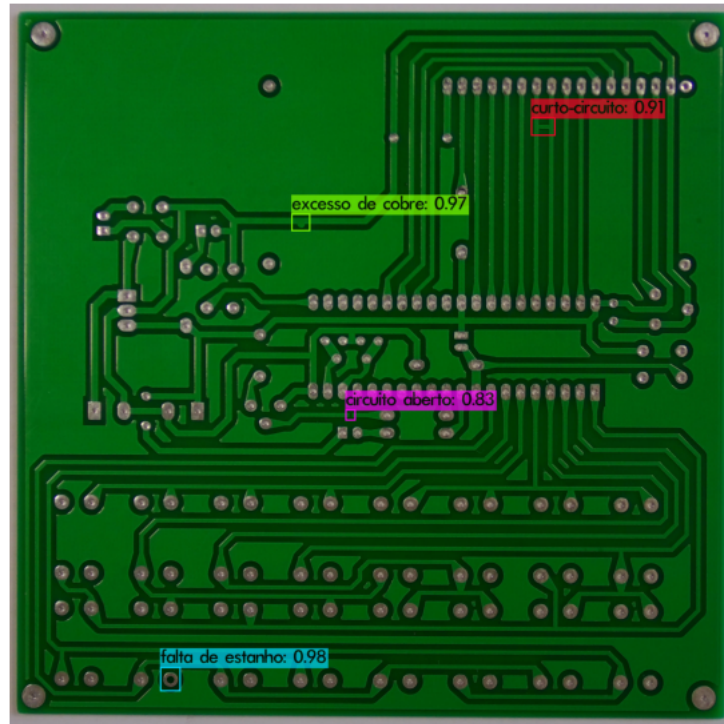
Figura 31 – Resultado de predição para imagem com defeito, teste 1.
