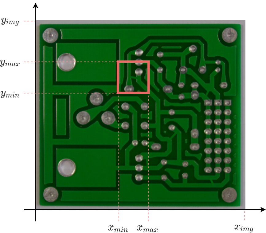
Figura 26 – Anotações das caixas delimitadoras do dataset HRIPCB.
