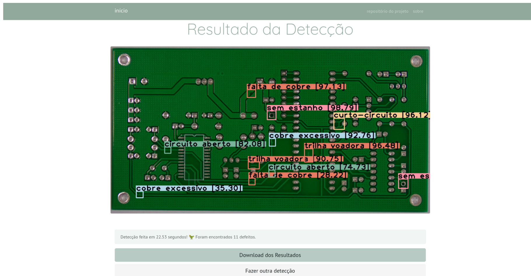
Figura 40 – Tela da Interface de Aplicação para imagem com detecções.
