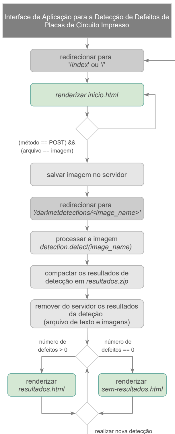
Figura 37 – Fluxograma da detecção de defeitos de placas de circuito impresso dentro da interface de aplicação proposta.
