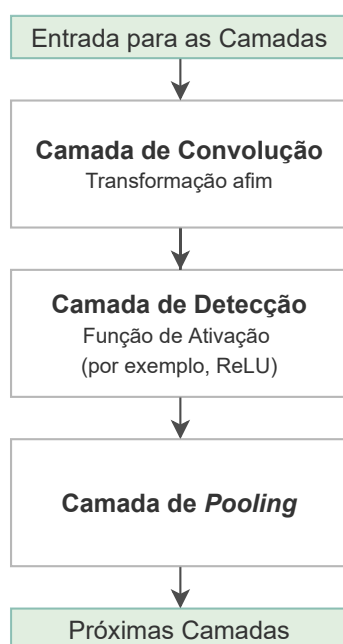
Figura 15 – Componentes de uma rede neural convolucional típica.
