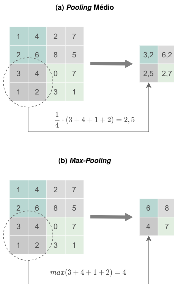
Figura 18 – Exemplos de funções utilizadas para operação de pooling .
