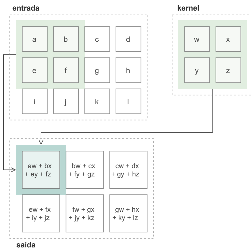
Figura 16 – Exemplo de convolução entre dois vetores bidimensionais.
