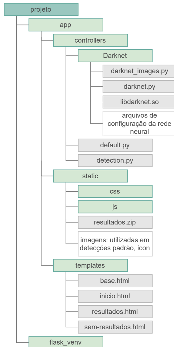
Figura 36 – Estrutura da interface de aplicação proposta.
