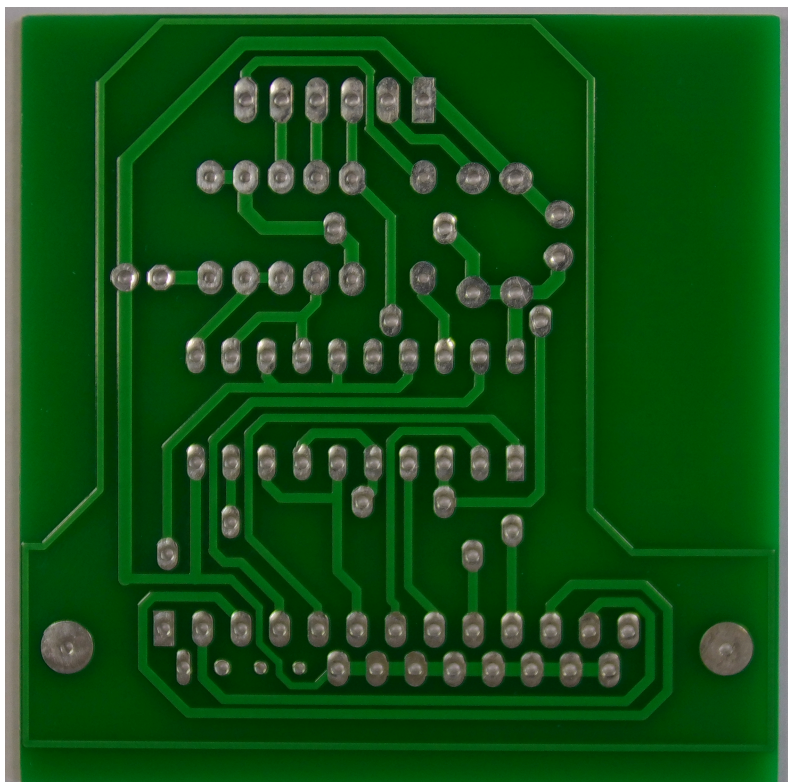
Figura 50 – PCI Número 11 do conjunto de dados HRIPCB.
