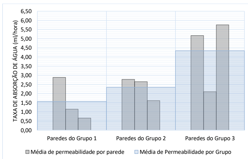
Figura 24 – Permeabilidades de água médias dos grupos de paredes.
