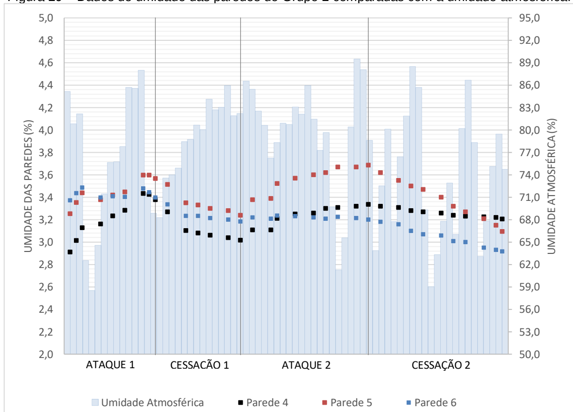
Figura 29 – Dados de umidade das paredes do Grupo 2 comparadas com a umidade atmosférica.
