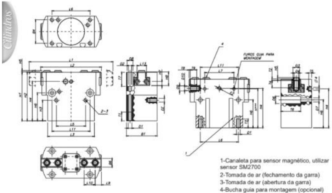
Figura 12 – Detalhamento dimensional da garra axial selecionada
