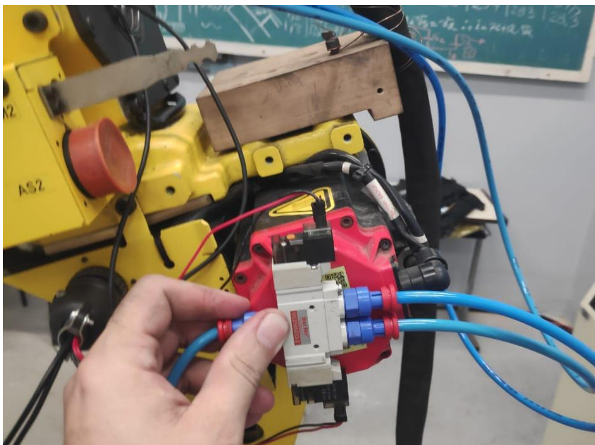
Figura 23 - Eletroválvula
