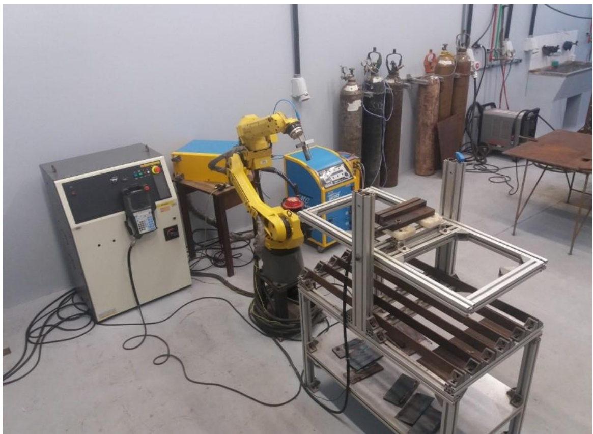
Figura 2 - Célula de soldagem robotizada do IFSC
