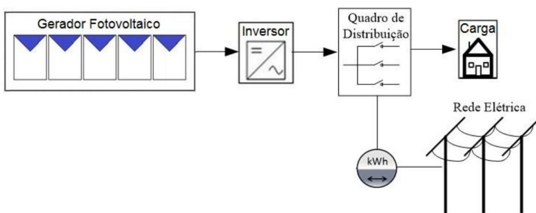
Figura 5 – Sistema conectado à rede
