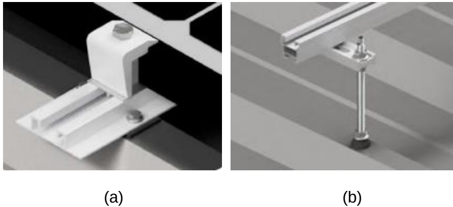
Figura 10 – Fixação em telhas metálicas
