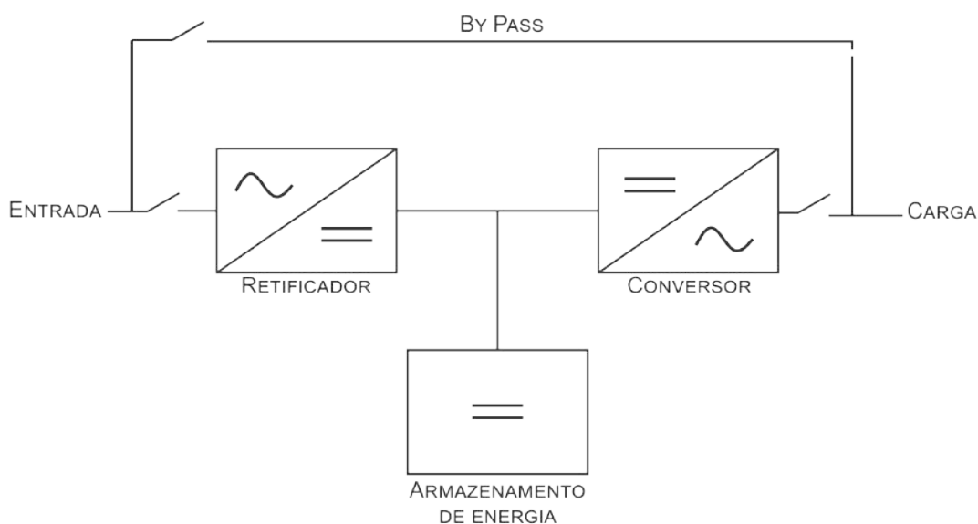
Figura 3 – Diagrama de blocos típico de funcionamento do UPS.
