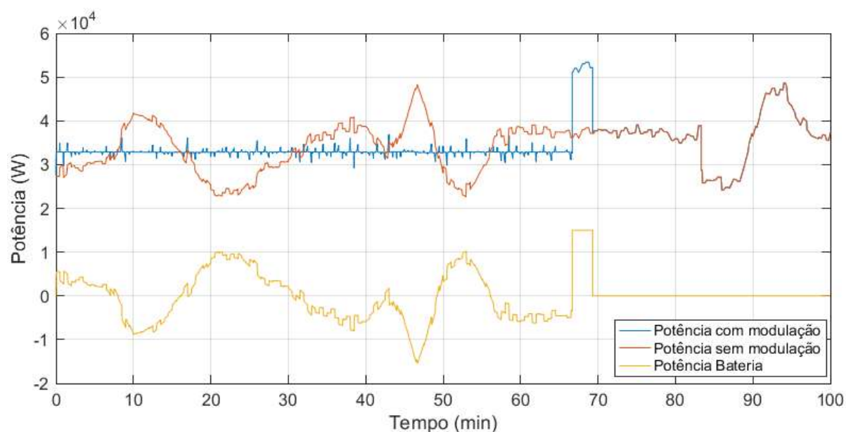
Figura 58 – Potência demandada da rede elétrica nos cenários com e sem modulação de corrente, com a mesma dinâmica da carga de TI e retorno ao estado inicial da carga da bateria.
