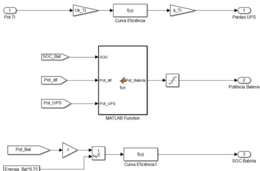
Figura 52 – Modelo do UPS em operação para auxílio à modulação de carga.
