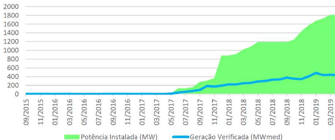
Figura 88 – Evolução da geração e potência instalada de usinas solares no SIN.
