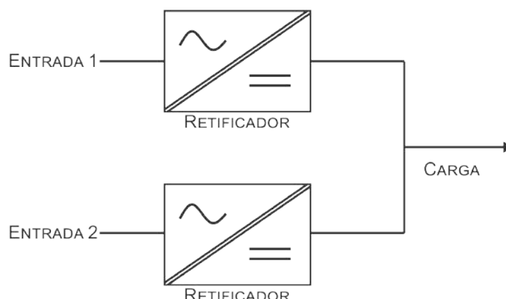
Figura 4 – Diagrama de blocos de funcionamento de uma fonte redundante.
