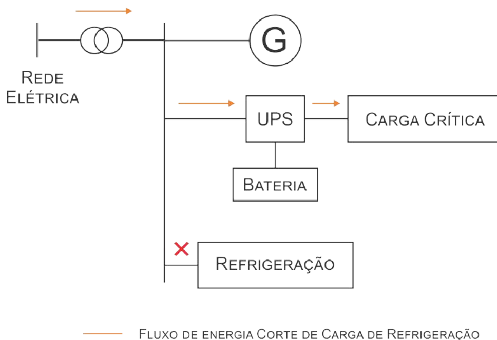
Figura 46 – Representação do fluxo de energia para o cenário corte de carga de refrigeração.
