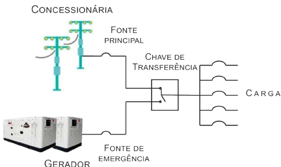
Figura 17 – Esquemático de funcionamento de uma chave de transferência automática.
