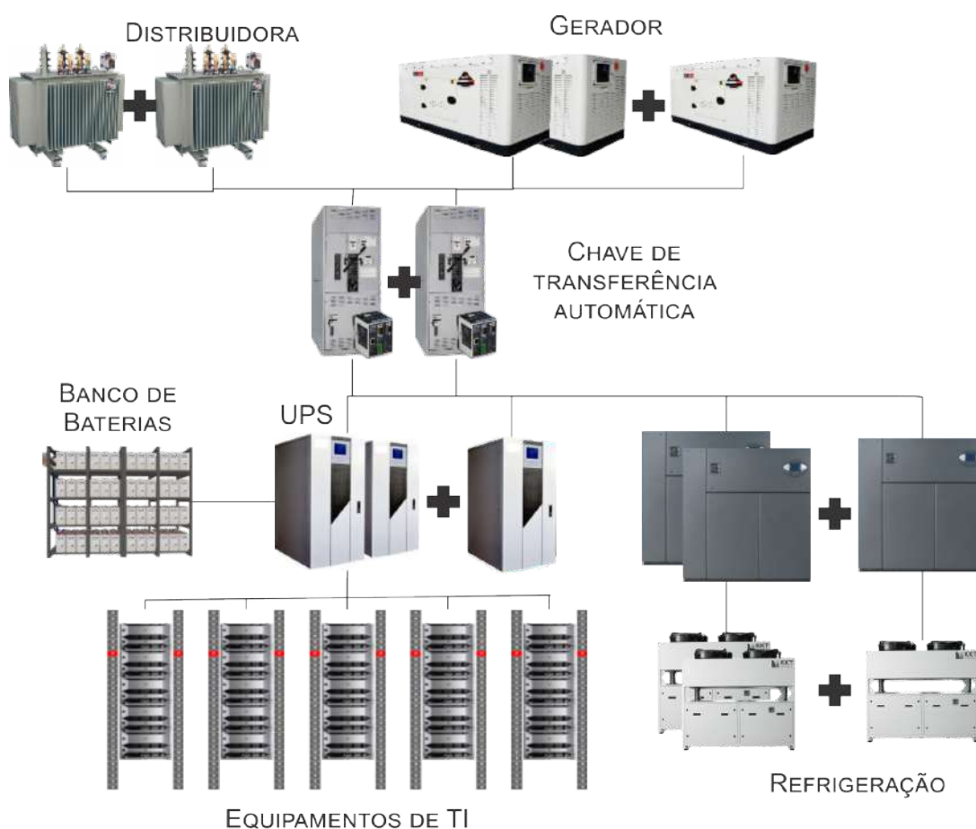
Figura 7 – Esquemático da arquitetura de um data center tier II.
