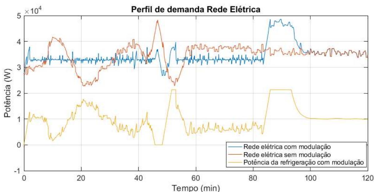
Figura 67 – Demanda de carga imposta a rede elétrica com e sem modulação de carga pelo sistema de refrigeração e potência aplicada ao sistema de refrigeração.
