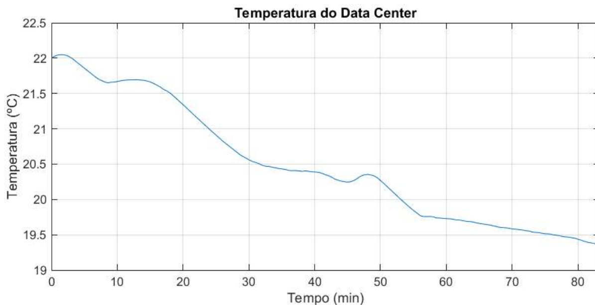
Figura 65 – Dinâmica da temperatura com modulação de carga pela refrigeração.
