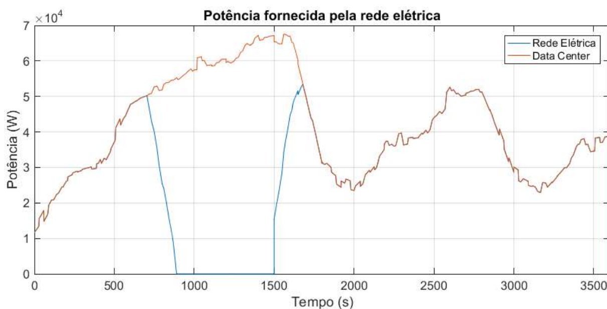
Figura 37 – Simulação do modelo do grupo moto gerador apresentada da perspectiva da rede elétrica.
