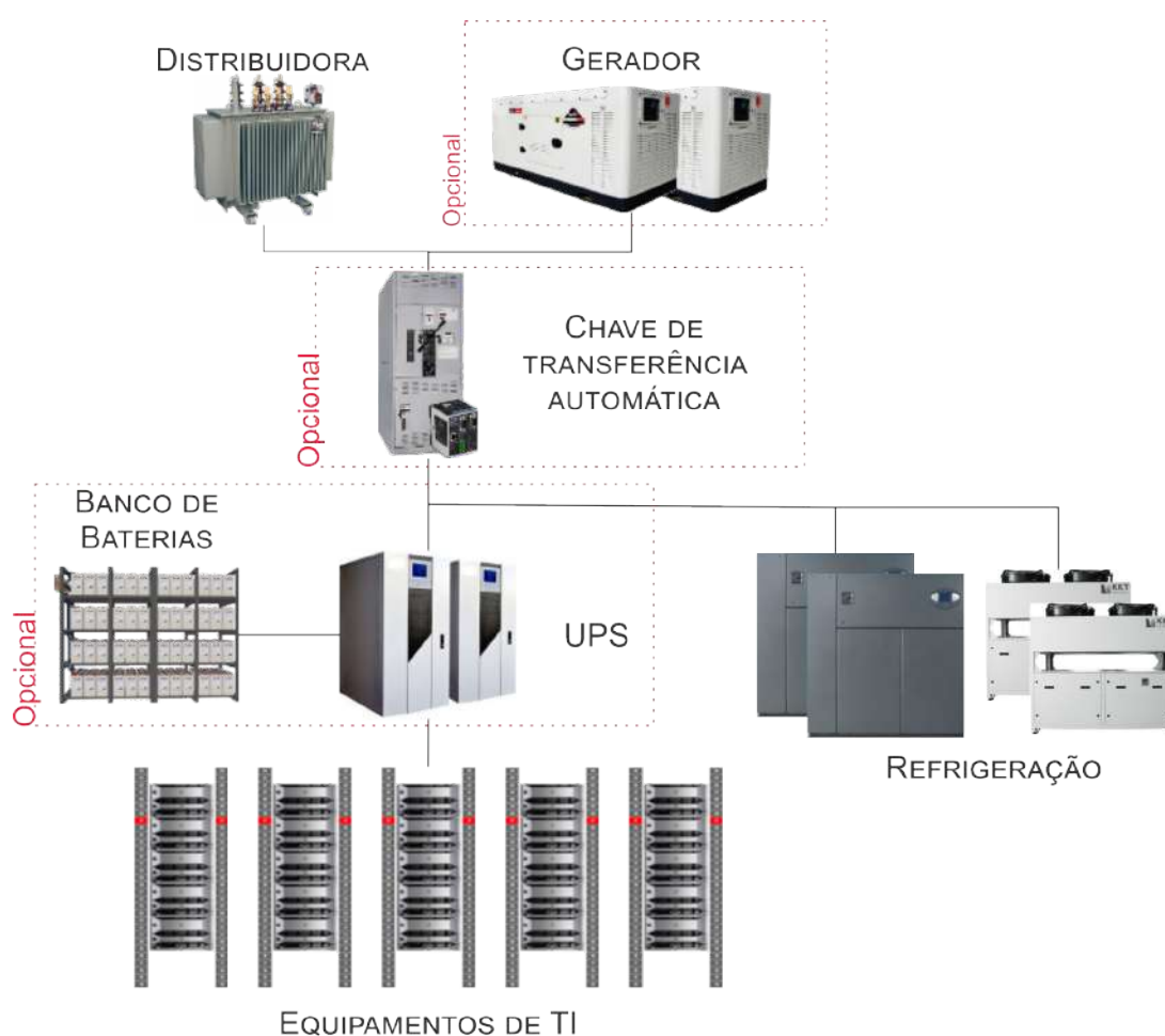
Figura 6 – Esquemático da arquitetura de um data center tier I.
