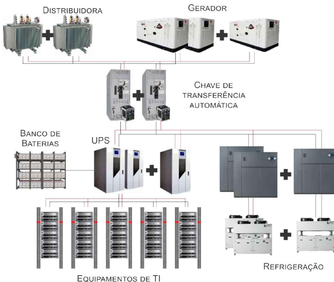
Figura 8 – Esquemático da arquitetura de um data center tier III.
