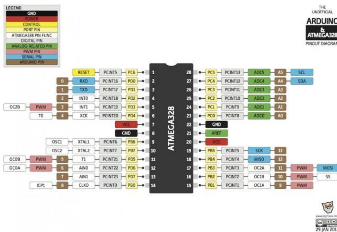
Figura 41 - Diagrama de portas do ATMEGA328P
