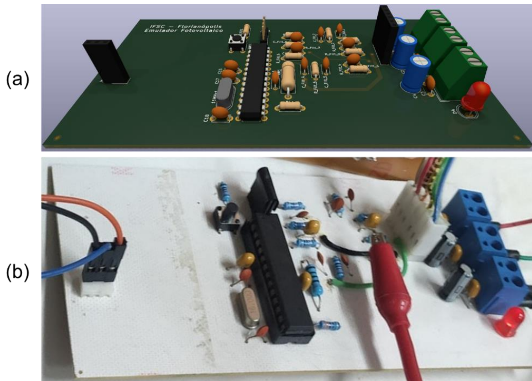
Figura 28 – (a) Representação em 3D da placa de comando projetada e (b) placa de comando após a montagem dos componentes eletrônicos
