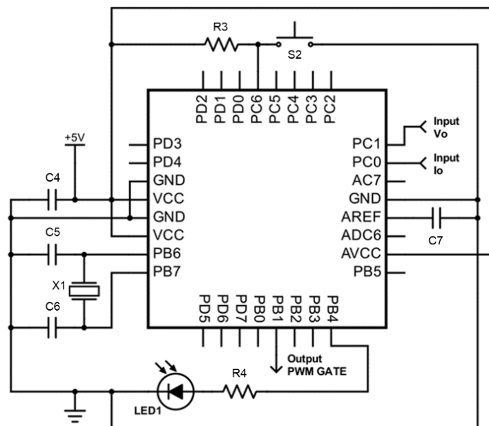
Figura 27 - Diagrama da placa de comando projetada
