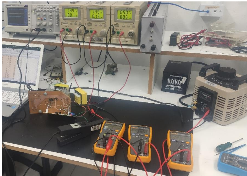
Figura 31 - Realização de ensaios no emulador fotovoltaico
