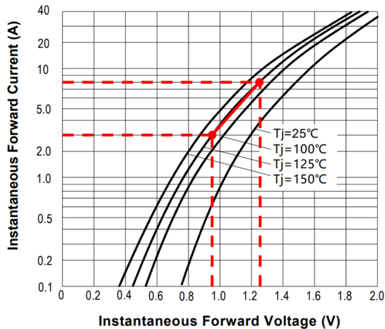
Figura 16 - Linearização da curva IV em 125°C do diodo MUR1660
