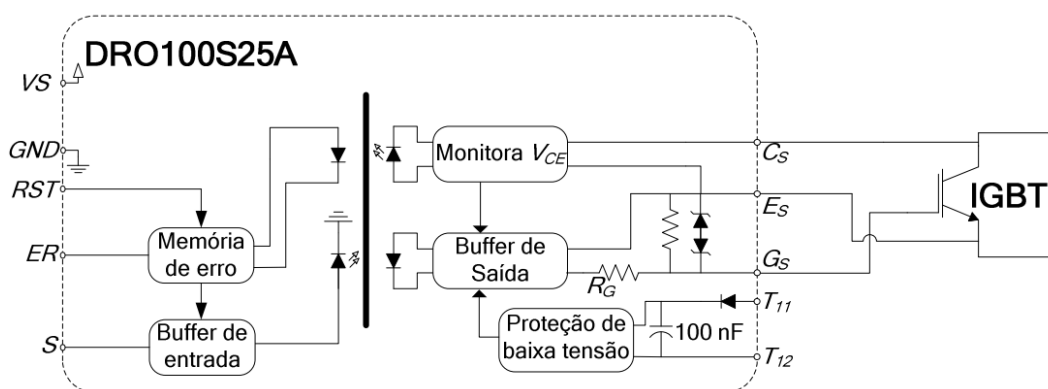
Figura 25 - Esquemático de funcionamento do driver isolador DRO100S25A
