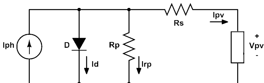
Figura 9 – Modelo equivalente de uma célula fotovoltaica
