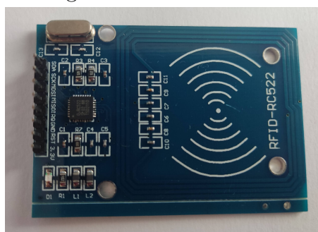
Figura 11 – Leitor RFID
