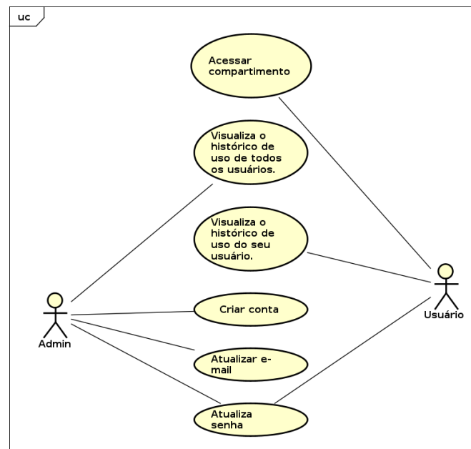
Figura 14 – Casos de Uso do servidor
