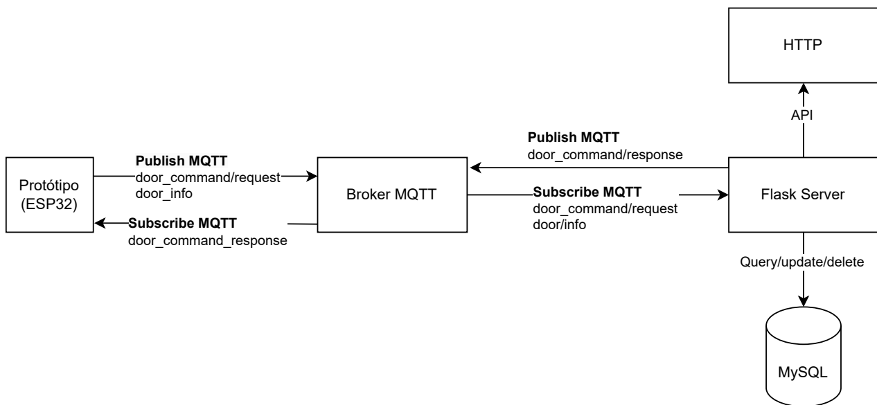
Figura 13 – Fluxo da comunicação no servidor
