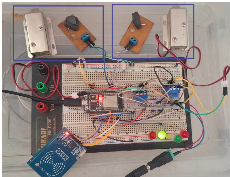
Figura 18 – Protótipo
