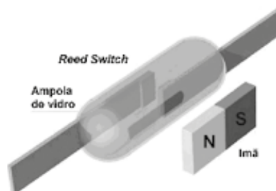
Figura 3 – Sensor de Proximidade Magnético
