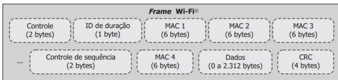
Figura 7 – Quadro de transmissão Wi-Fi
