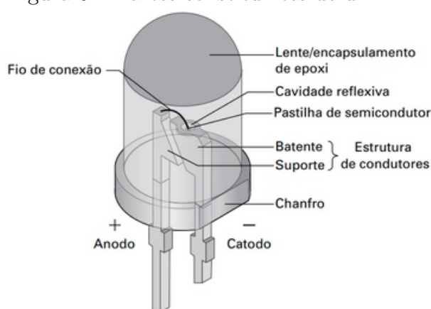
Figura 6 – Partes constituintes de um LED
