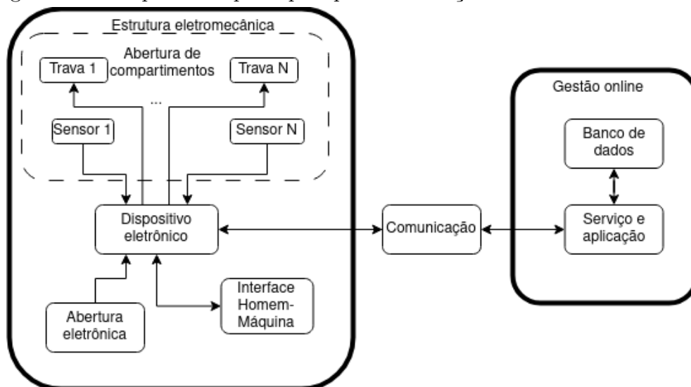
Figura 1 – Componentes principais para construção de armários eletrônicos
