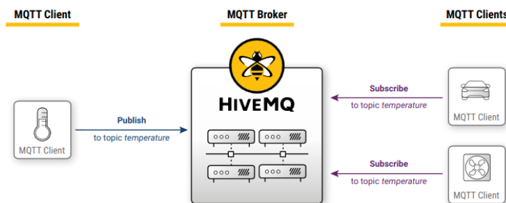
Figura 8 – Arquitetura Publish/Subscribe
