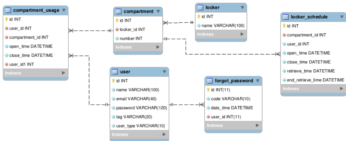
Figura 12 – Modelagem do Banco de Dados da aplicação.
