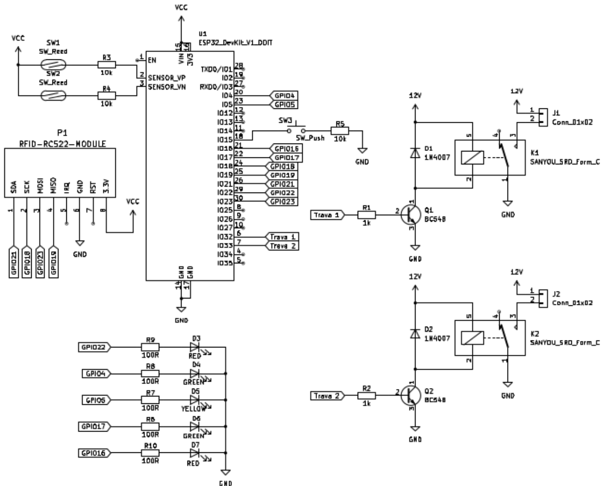
Figura 17 – Esquemático eletrônico
