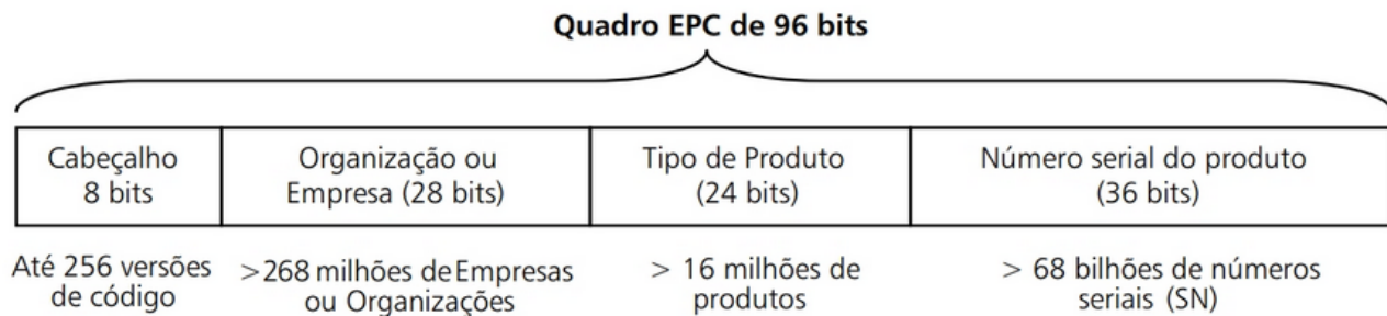
Figura 5 – Estrutura de um quadro EPC
