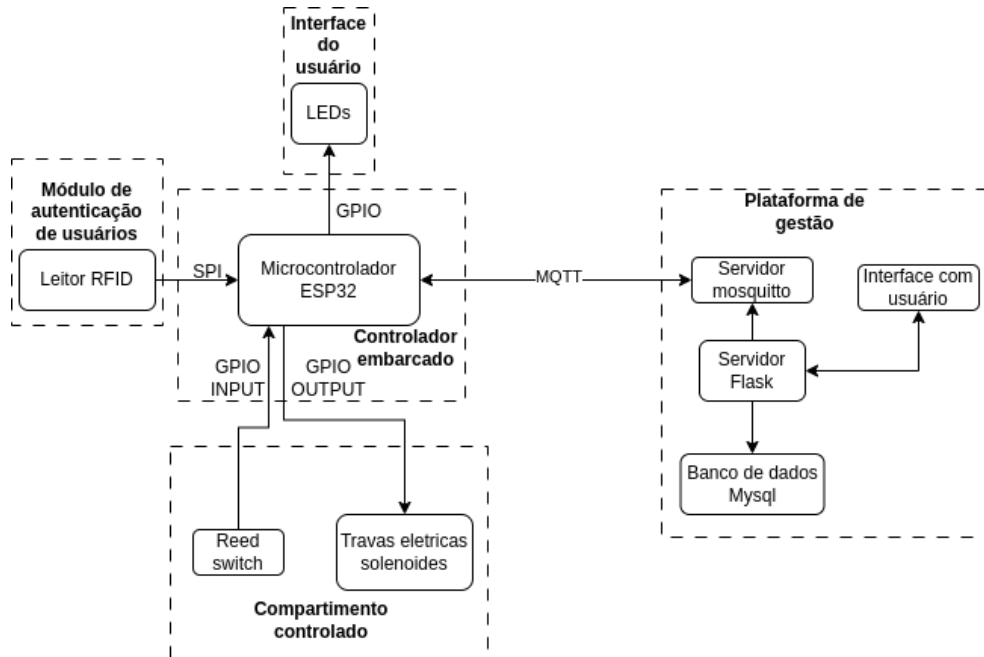
Figura 10 – Componentes da solução de guarda-volumes inteligentes com auditoria
