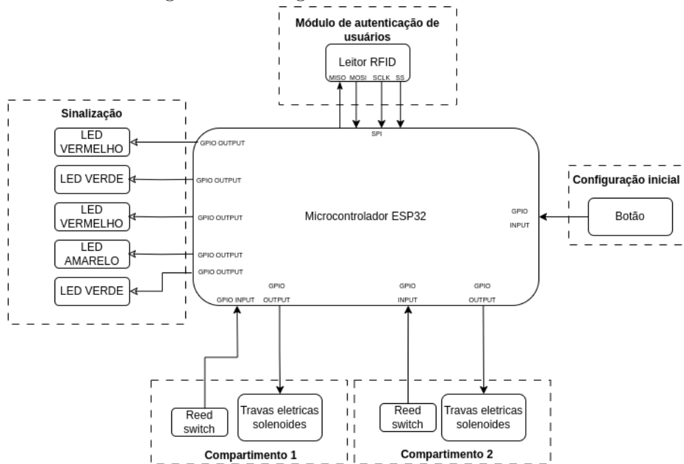
Figura 16 – Diagrama de blocos de hardware
