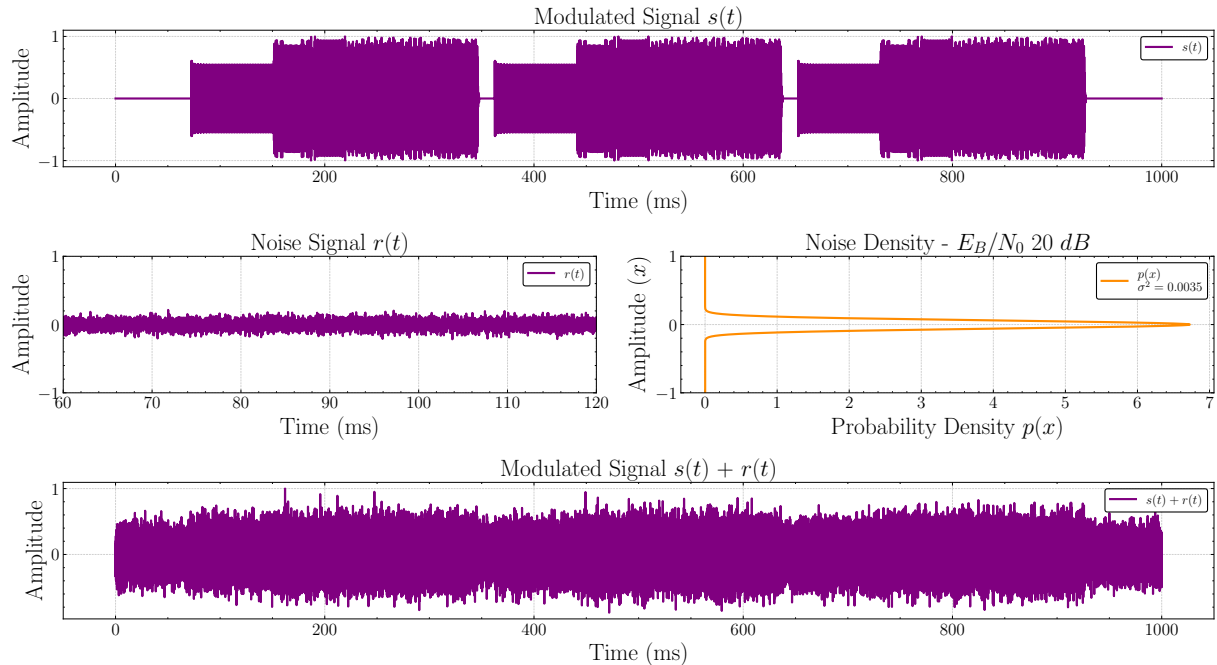
Figura 25 – Adição de ruído ao canal
