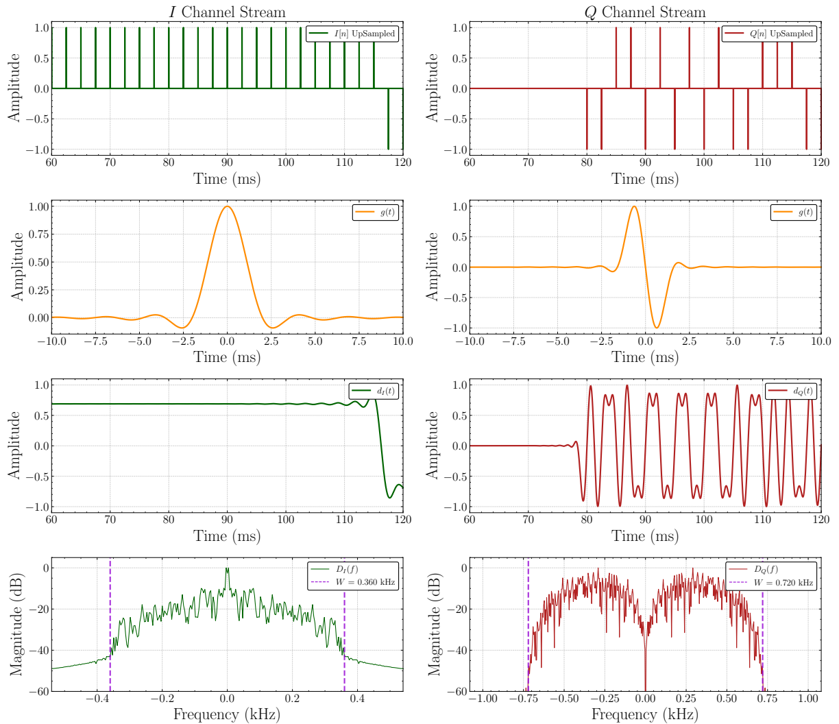
Figura 21 – Modulação de pulso dos canais I e Q
