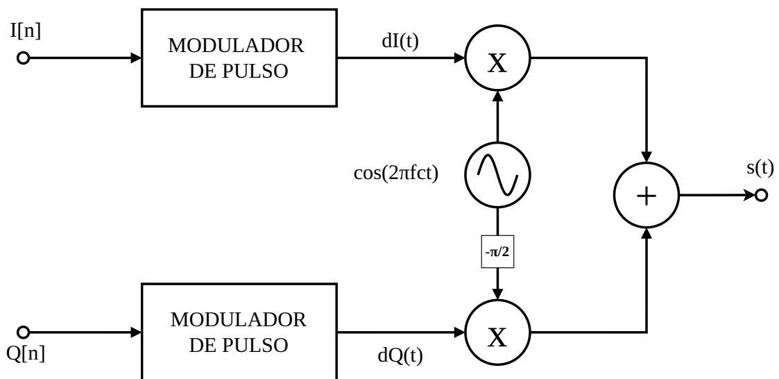
Figura 10 – Diagrama de blocos do modulador QPSK
