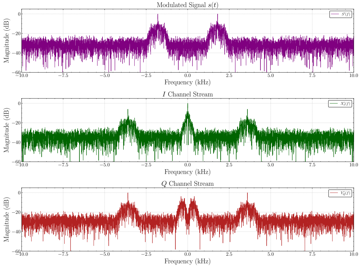
Figura 32 – Componentes I e Q após demodulação
