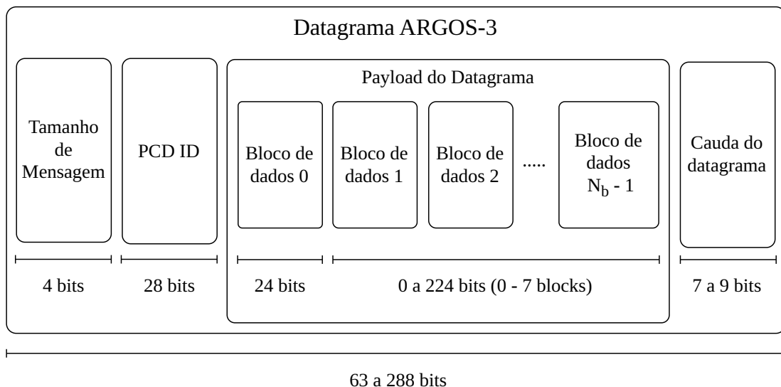
Figura 5 – Estrutura do datagrama ARGOS-3
