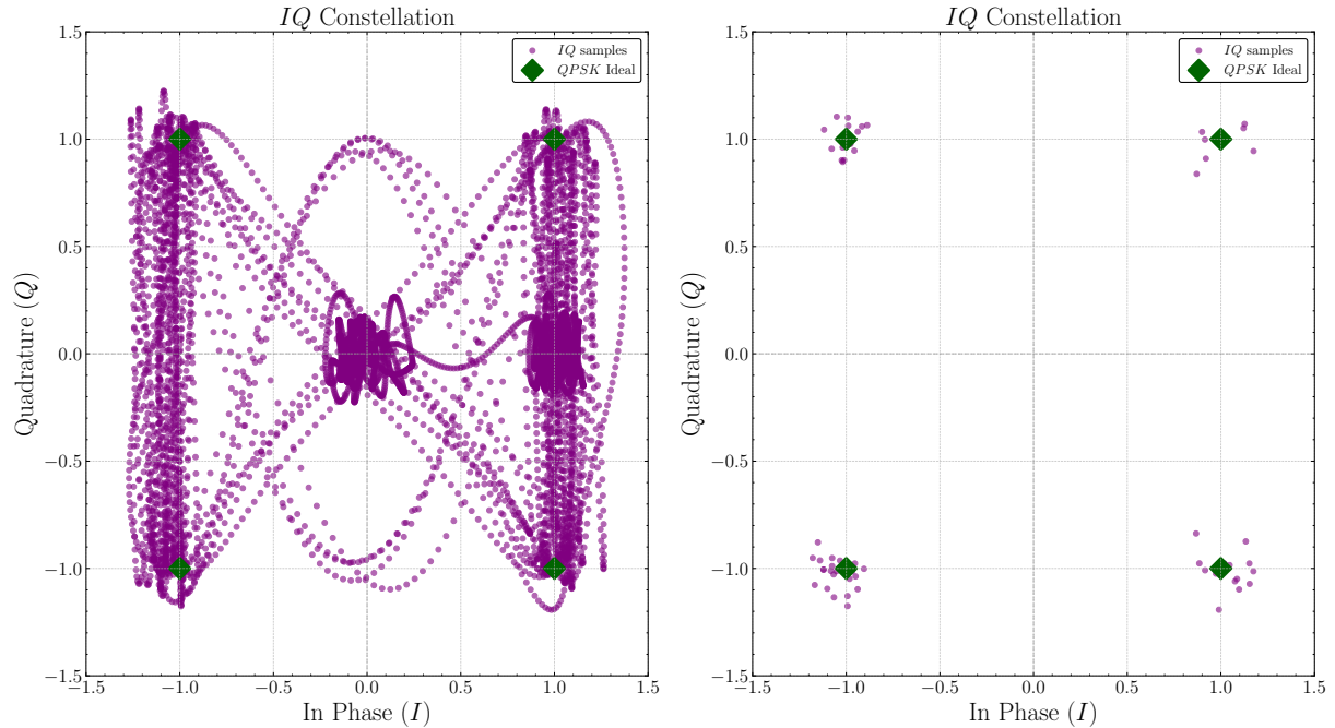
Figura 40 – Constelação dos canais I e Q filtrados e amostrados
