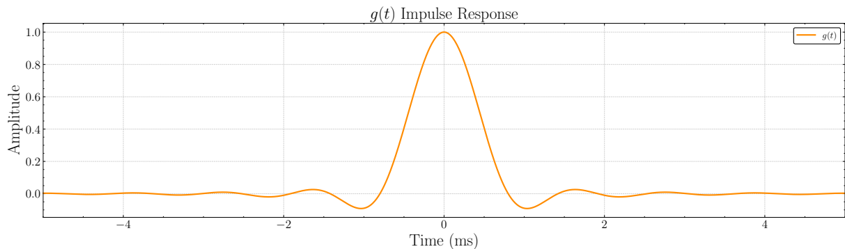
Figura 19 – Resposta ao impulso - Pulso RRC
