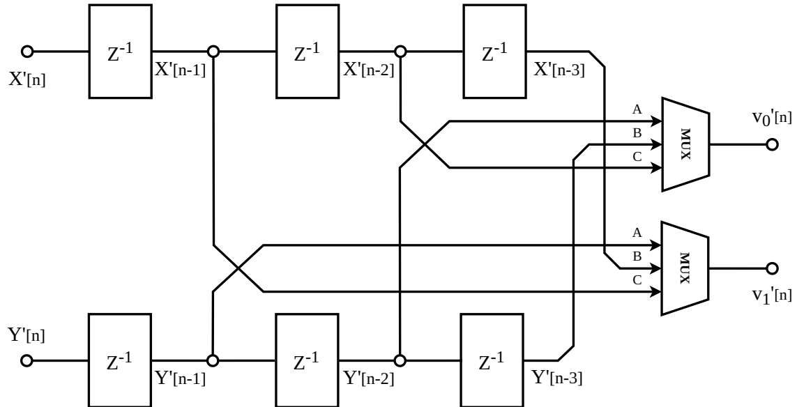
Figura 12 – Diagrama de blocos do Desembaralhador ARGOS-3
