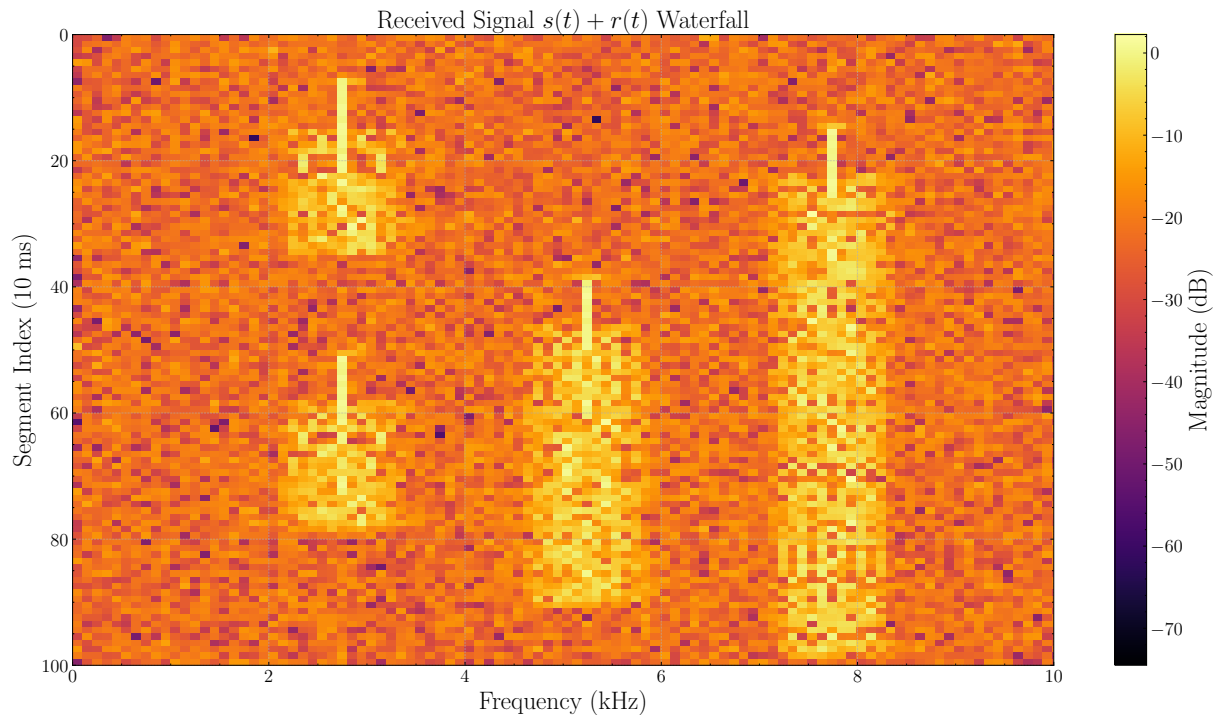
Figura 27 – Diagrama de waterfall do canal
