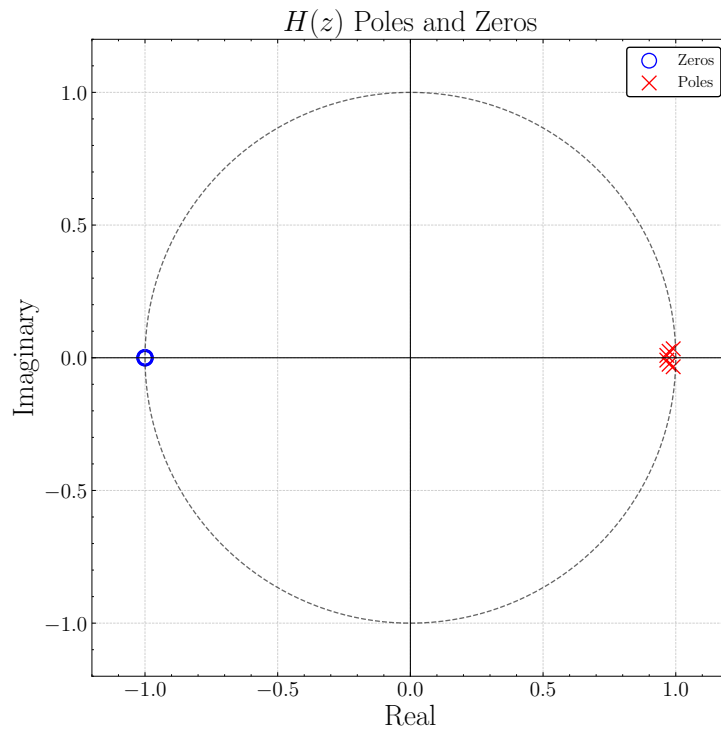
Figura 11 – Polos e zeros do filtro Passa Baixa
