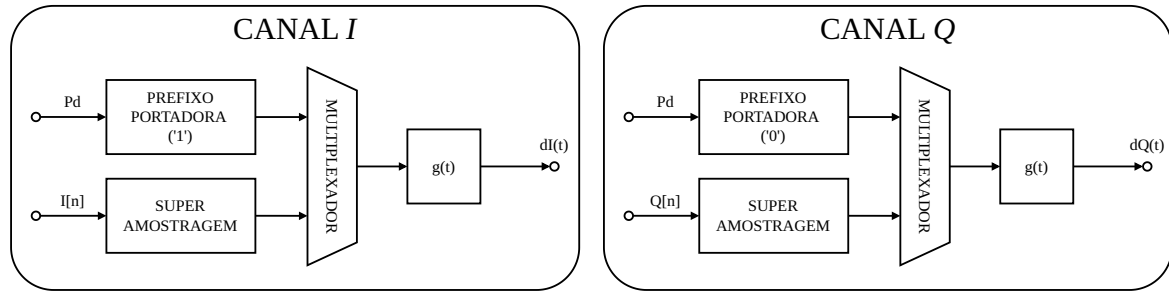
Figura 18 – Diagrama de blocos do modulador de pulso para os canais I e Q
