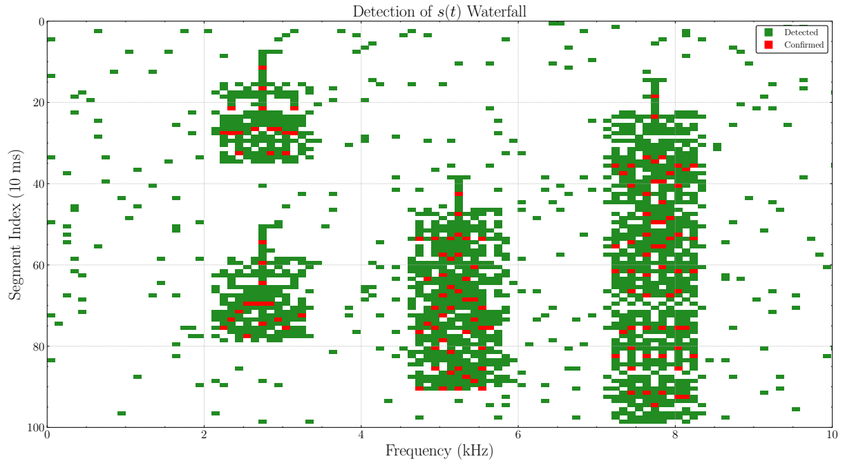
Figura 29 – Diagrama de waterfall de detecção do canal
