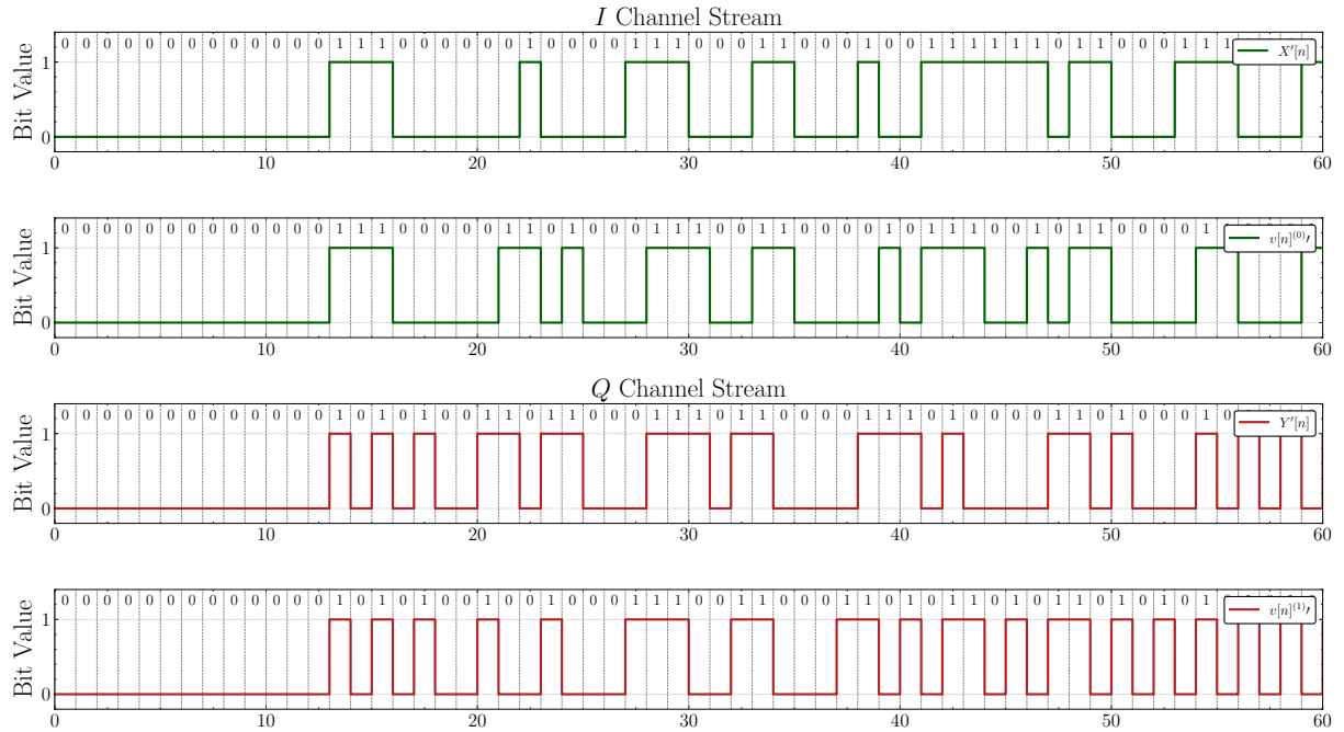
Figura 41 – Desembaralhamento dos canais I e Q
