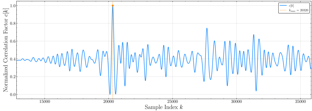
Figura 37 – Módulo de correlação entre I e Q e vetor de sincronismo
