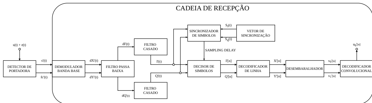
Figura 31 – Diagrama de blocos do receptor ARGOS-3
