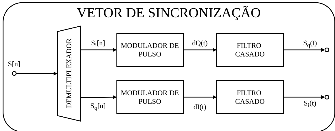
Figura 35 – Diagrama de blocos para montagem do vetor de sincronismo
