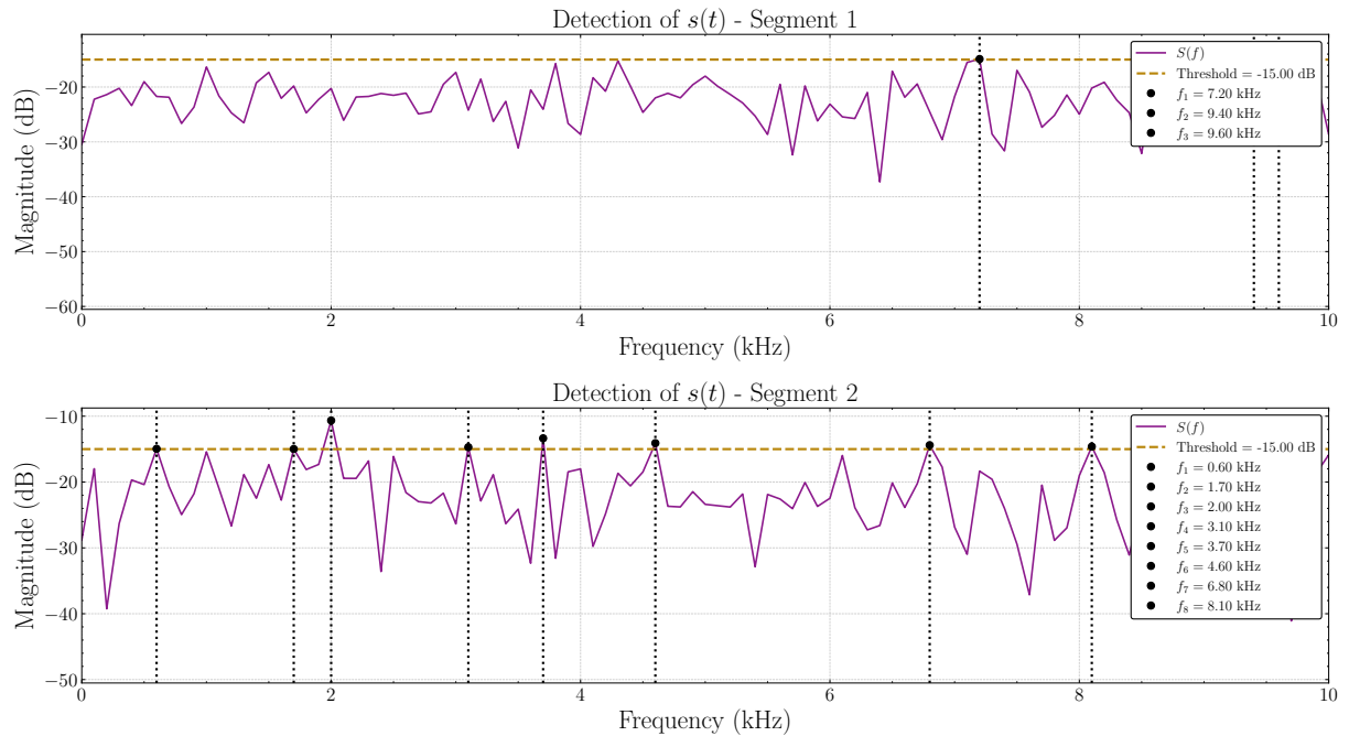
Figura 28 – Detecção de componentes no espectro com base em P_t
