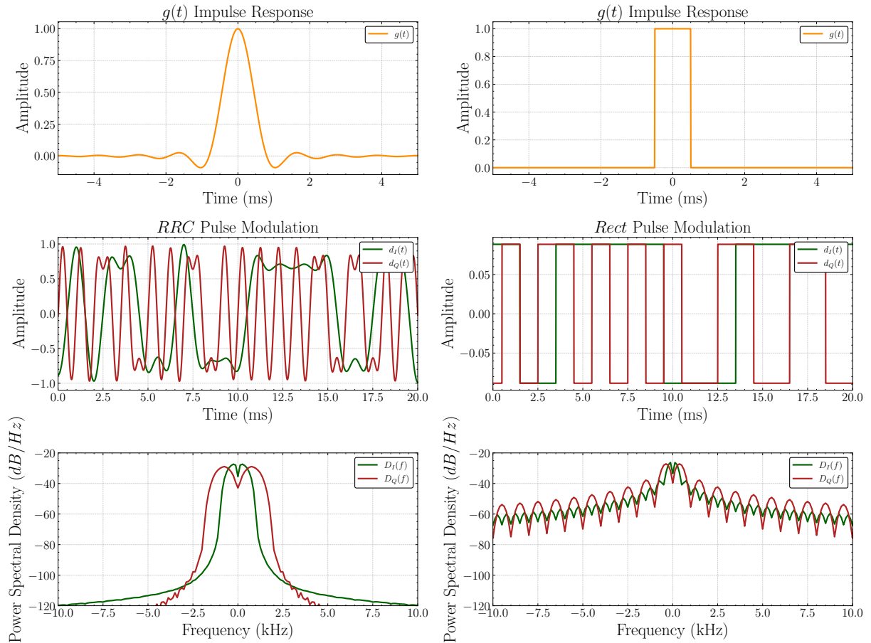
Figura 9 – Comparação entre modulação de pulso RRC e Rect
