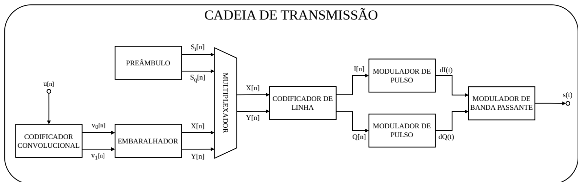
Figura 14 – Diagrama de blocos do transmissor ARGOS-3
