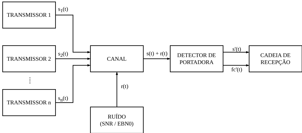
Figura 24 – Diagrama de blocos do canal
