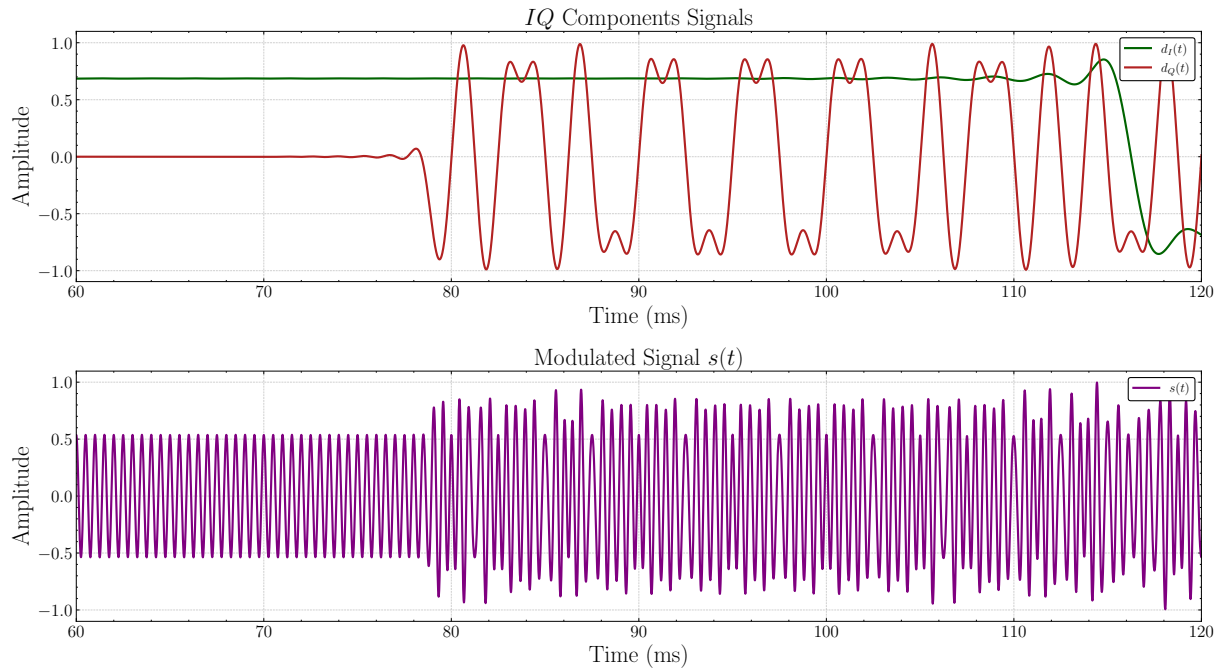
Figura 22 – Modulação em banda passante canais I e Q
