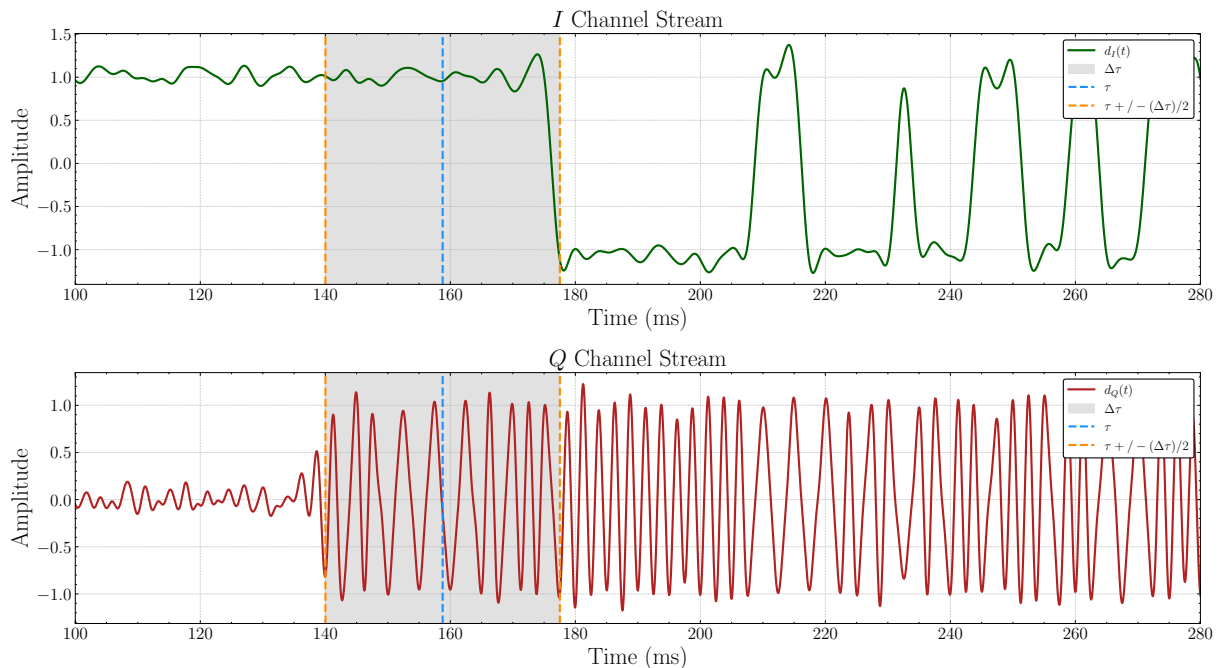
Figura 38 – Sincronização de I e Q com vetor de sincronismo
