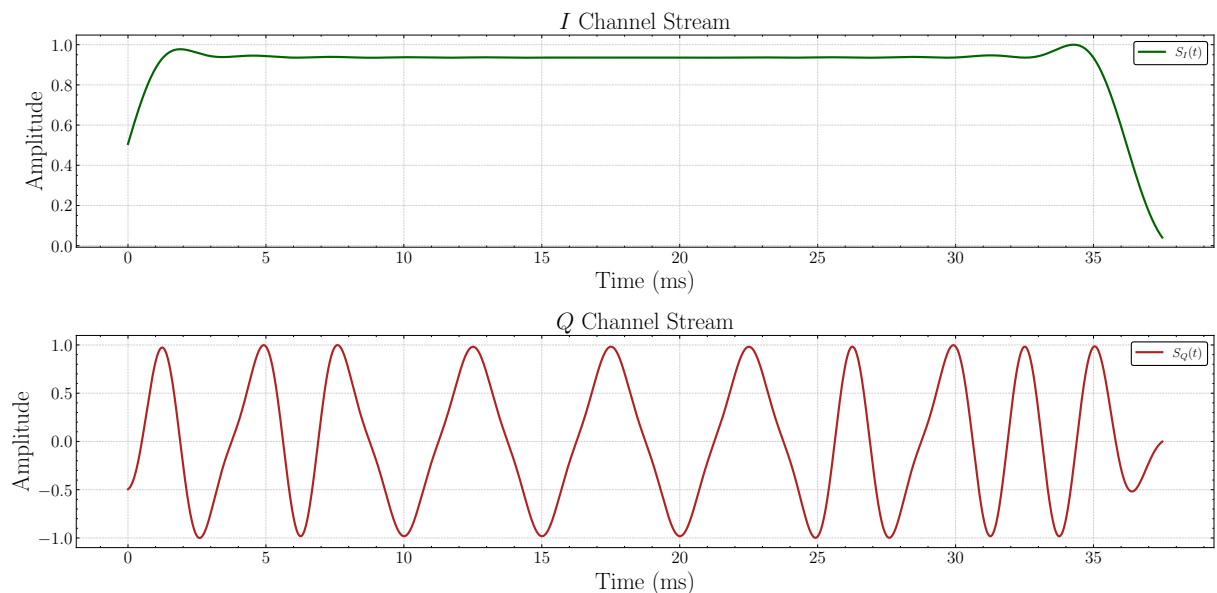
Figura 36 – Vetor de amostras esperadas para sincronismo com I e Q
