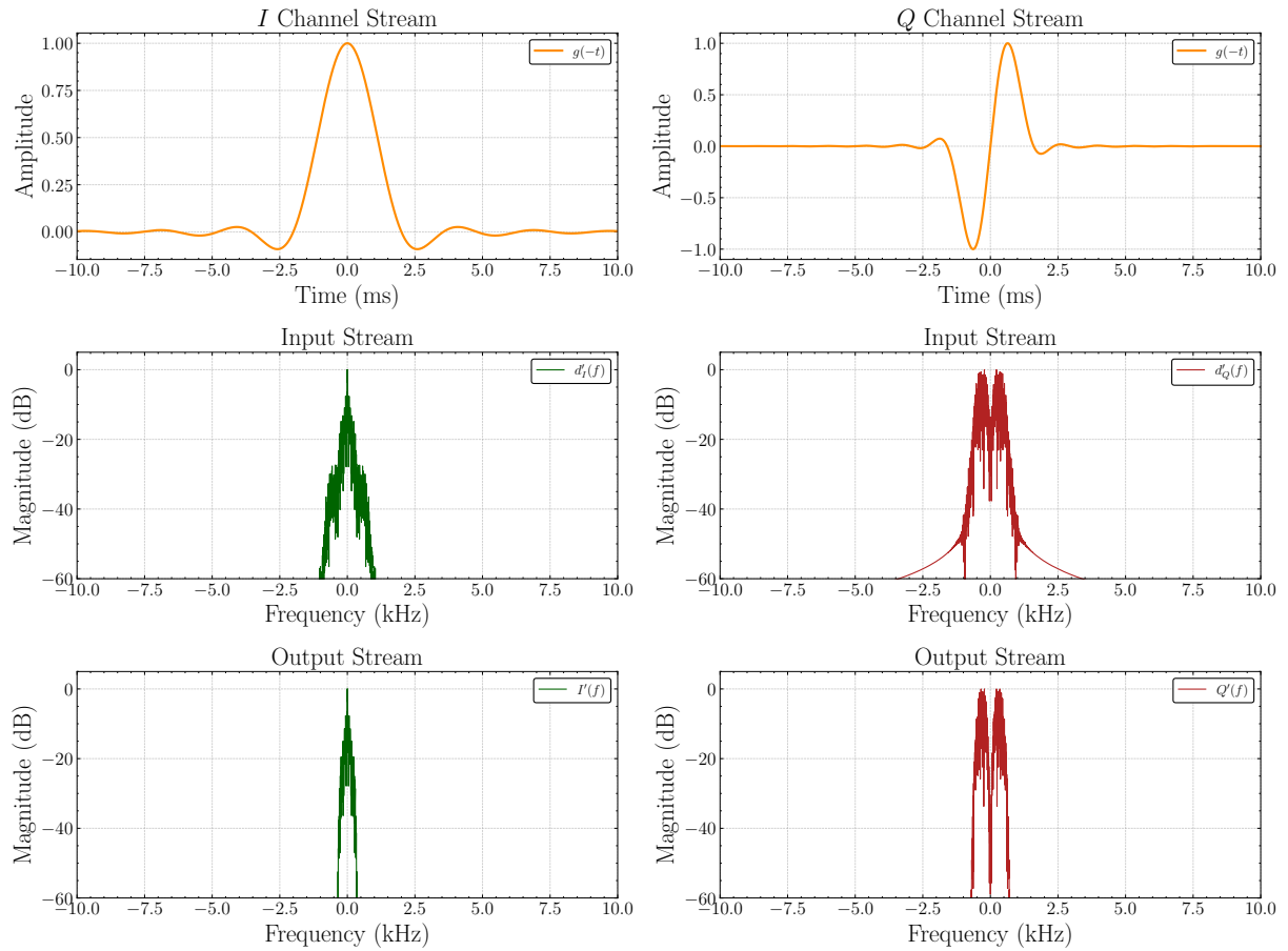
Figura 34 – Filtragem casada dos canais I e Q
