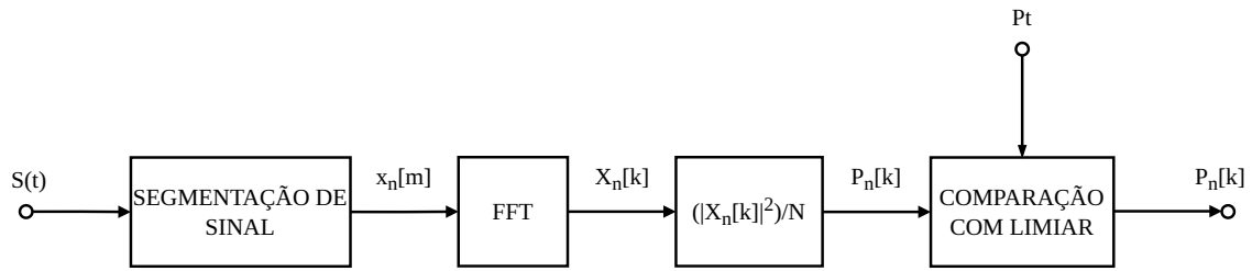
Figura 26 – Diagrama de blocos da detecção de portadora
