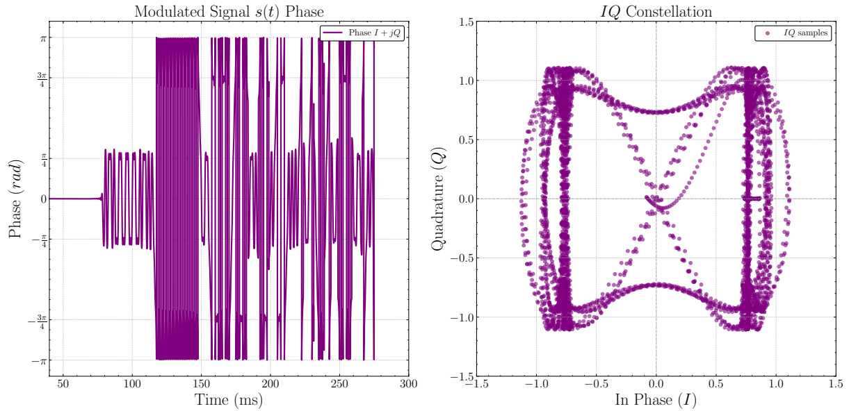
Figura 23 – Fase e Constelação do sinal modulado s(t)
