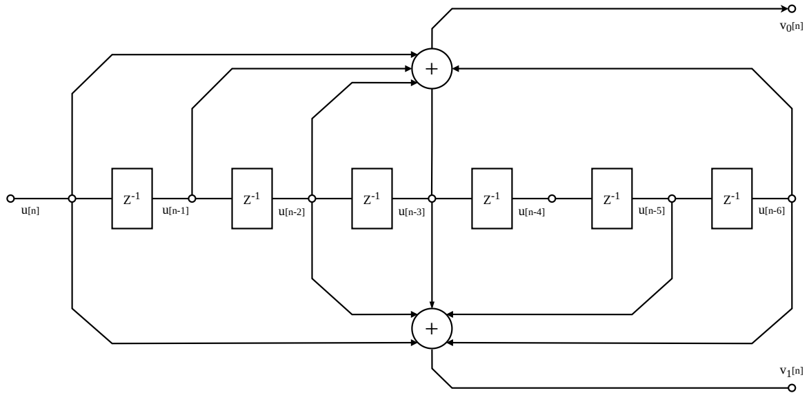
Figura 7 – Diagrama de blocos do codificador convolucional ARGOS-3
