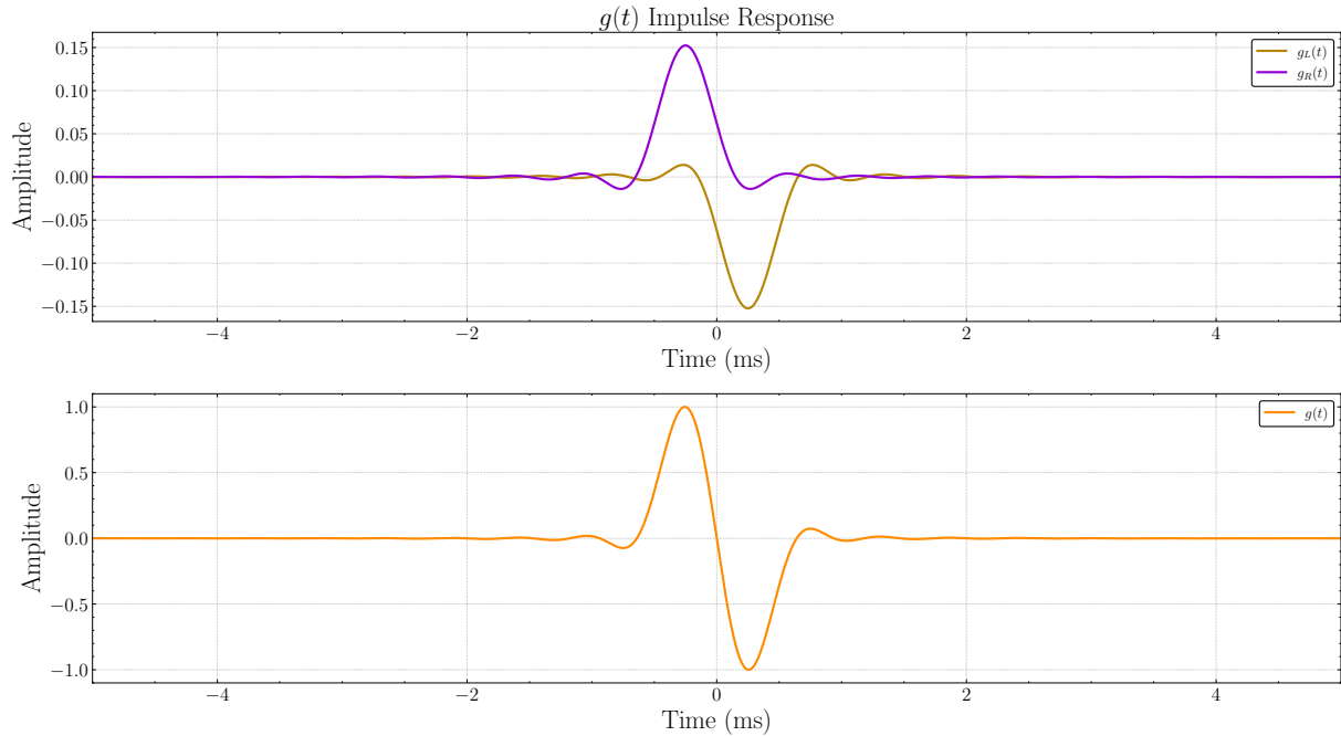
Figura 20 – Resposta ao impulso - Pulso Manchester
