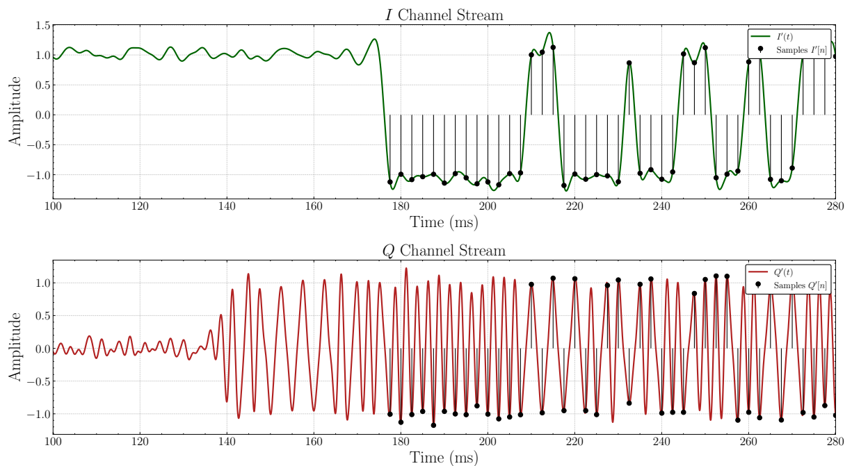
Figura 39 – Amostragem dos canais I e Q em T_b a partir de \tau
