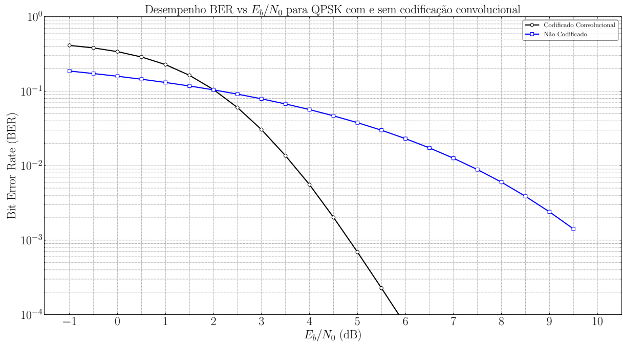
Figura 13 – Comparação de BER vs E_b/N_0 utilizando codificação convolucional
