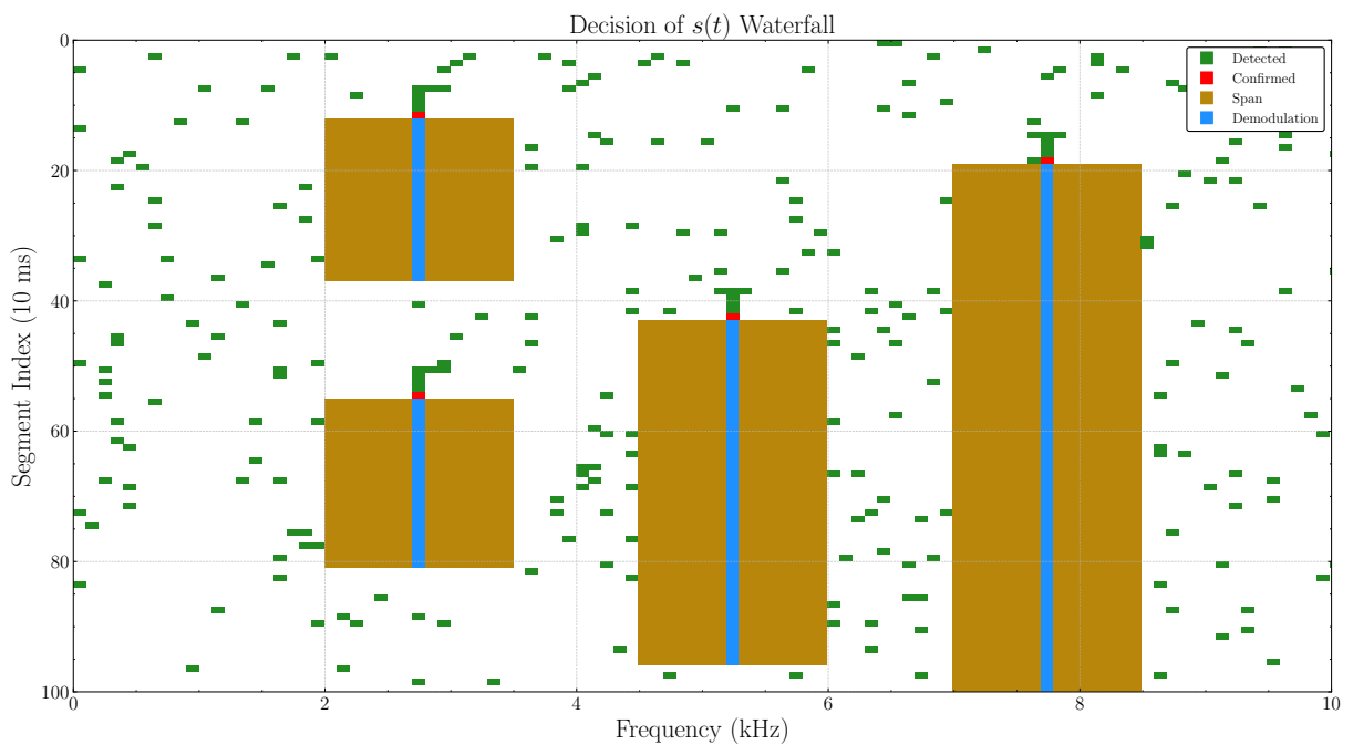
Figura 30 – Diagrama de waterfall de decisão do canal
