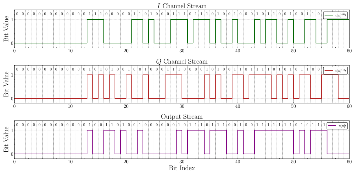
Figura 42 – Decodificação convolucional dos canais I e Q
