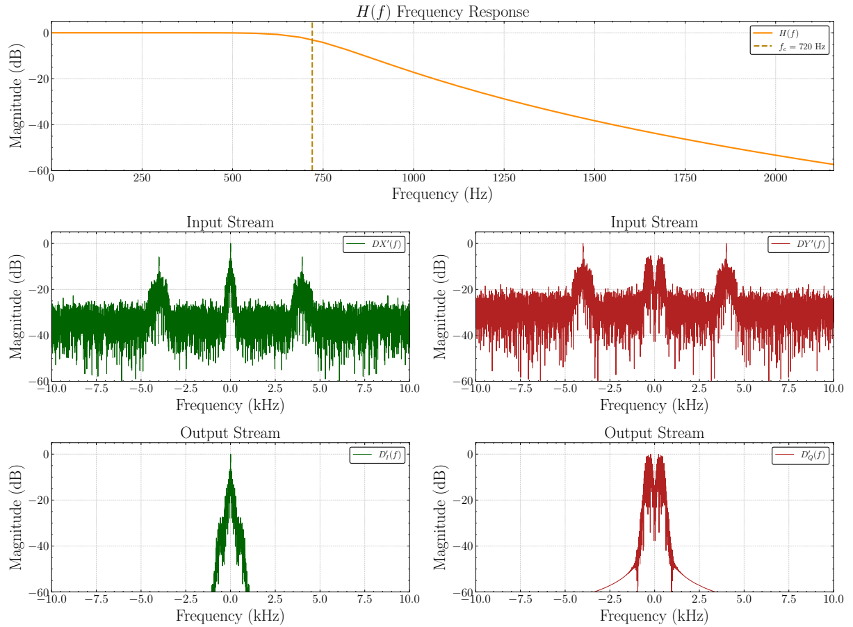
Figura 33 – Componentes I Q após filtragem passa baixa
