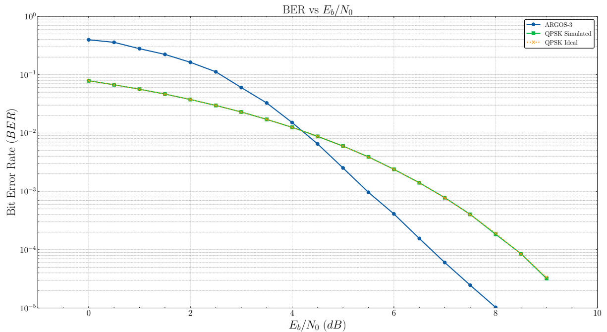
Figura 43 – Comparação BER vs SNR - ARGOS3 e QPSK
