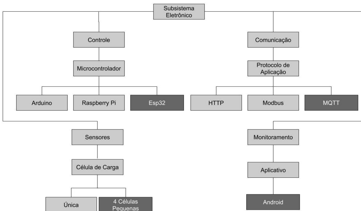
Figura 12 - Subsistema Eletrônico
