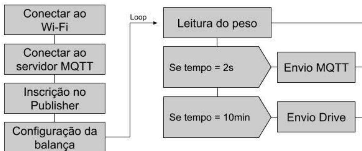
Figura 19 - Funcionamento do microcontrolador
