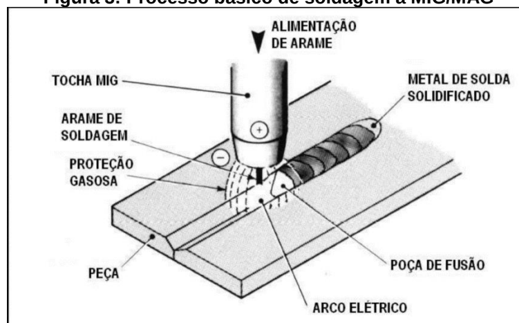
Figura 3: Processo básico de soldagem a MIG/MAG
