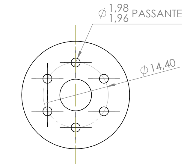
VISTA POSTERIOR
