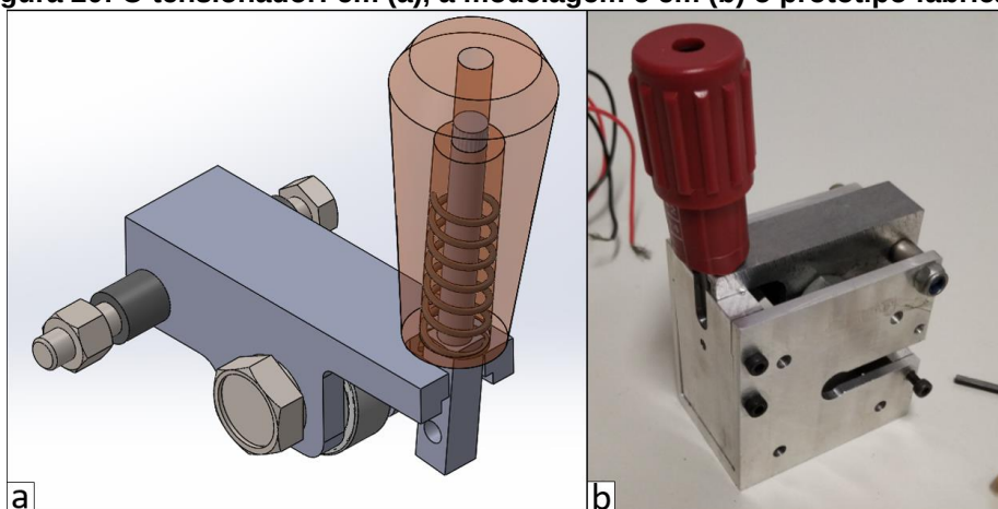
Figura 20: O tensionador: em (a), a modelagem e em (b) o protótipo fabricado
